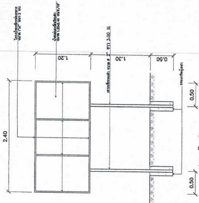
รูปตัดป้ายโครงการ not to scale
